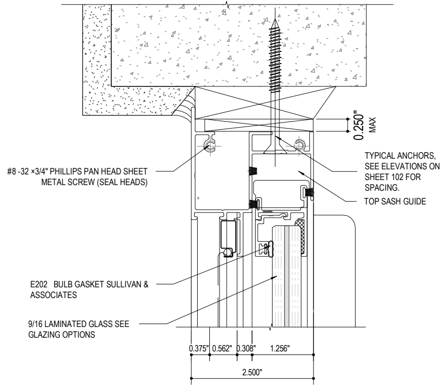
1 HEAD DETAIL THRU VENT N.T.S.
