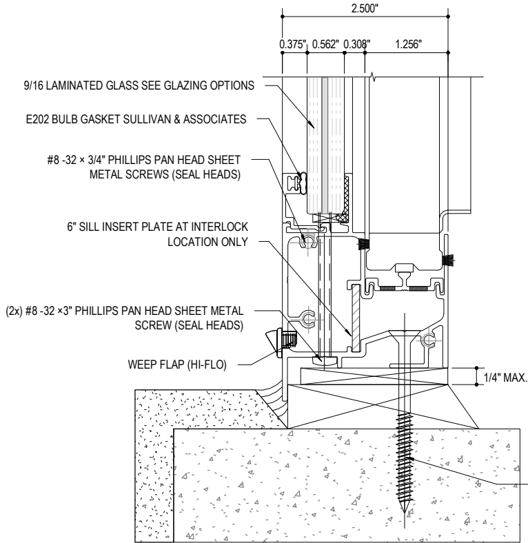
2 104 SILL DETAIL THRU FIX N.T.S.
