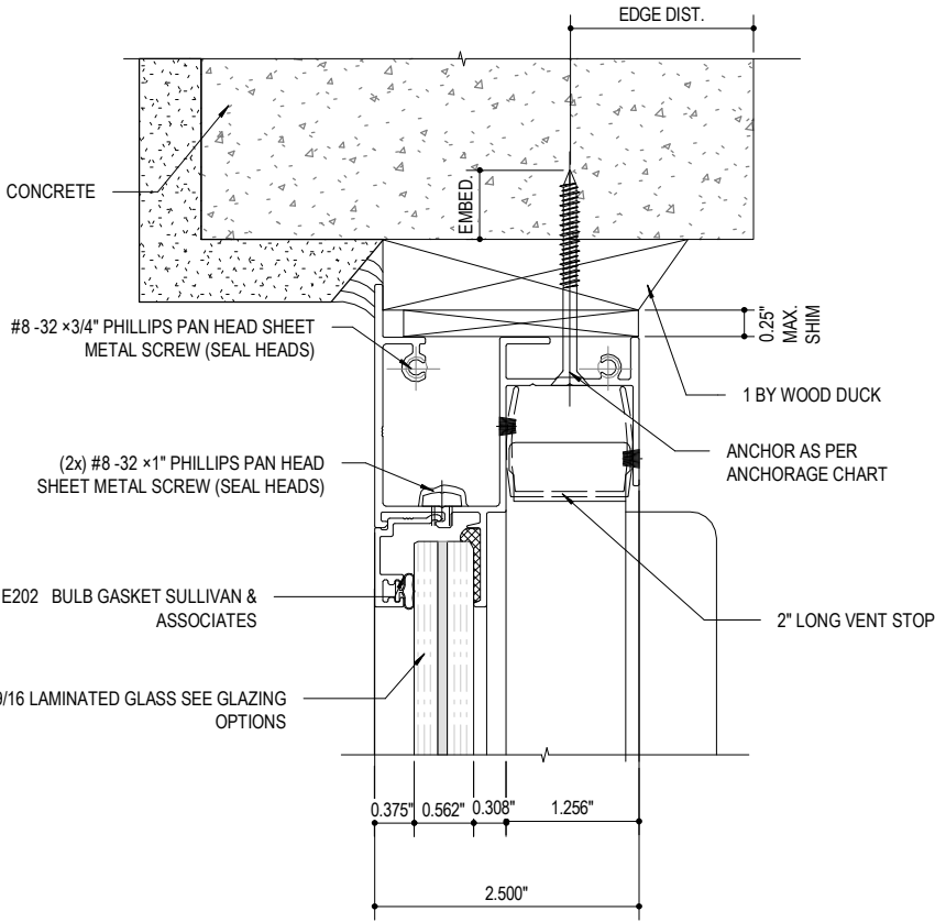
1 104 HEAD DETAIL THRU FIX N.T.S.
