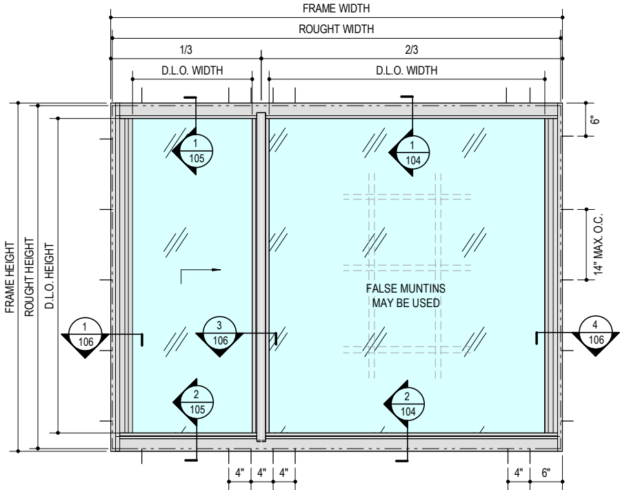
1 103 XO CONFIGURATION (1/3-2/3) N.T.S.
