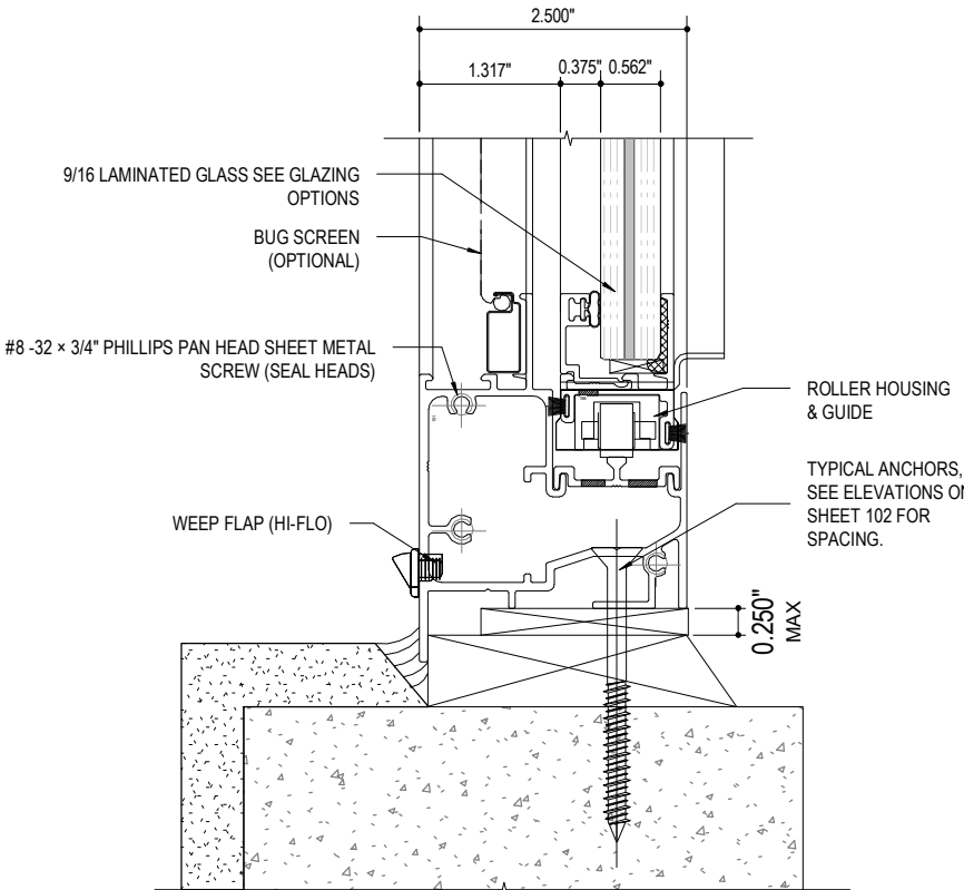
2 SILL DETAIL THRU VENT N.T.S.
