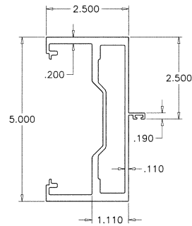
E3 DOOR JAMB Series 9000
