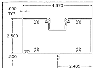
E1 DOOR HEADER Series 9000
