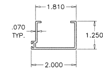
E18 CLOSURE DOOR STOP
