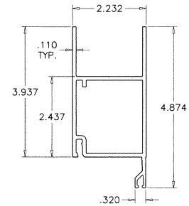
E4 TOP RAIL
