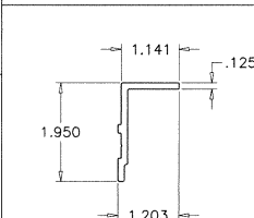
E14 LOCK BACK UP PLATE
